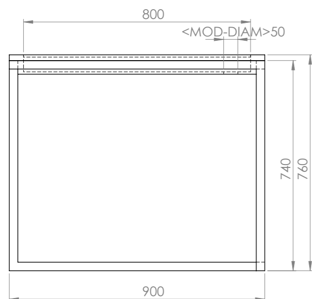
prerez B-B
