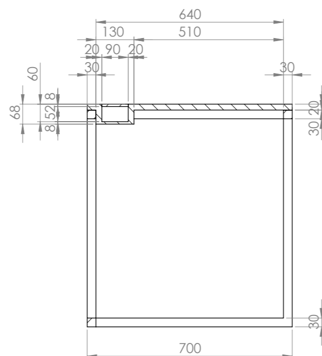
prerez A-A
