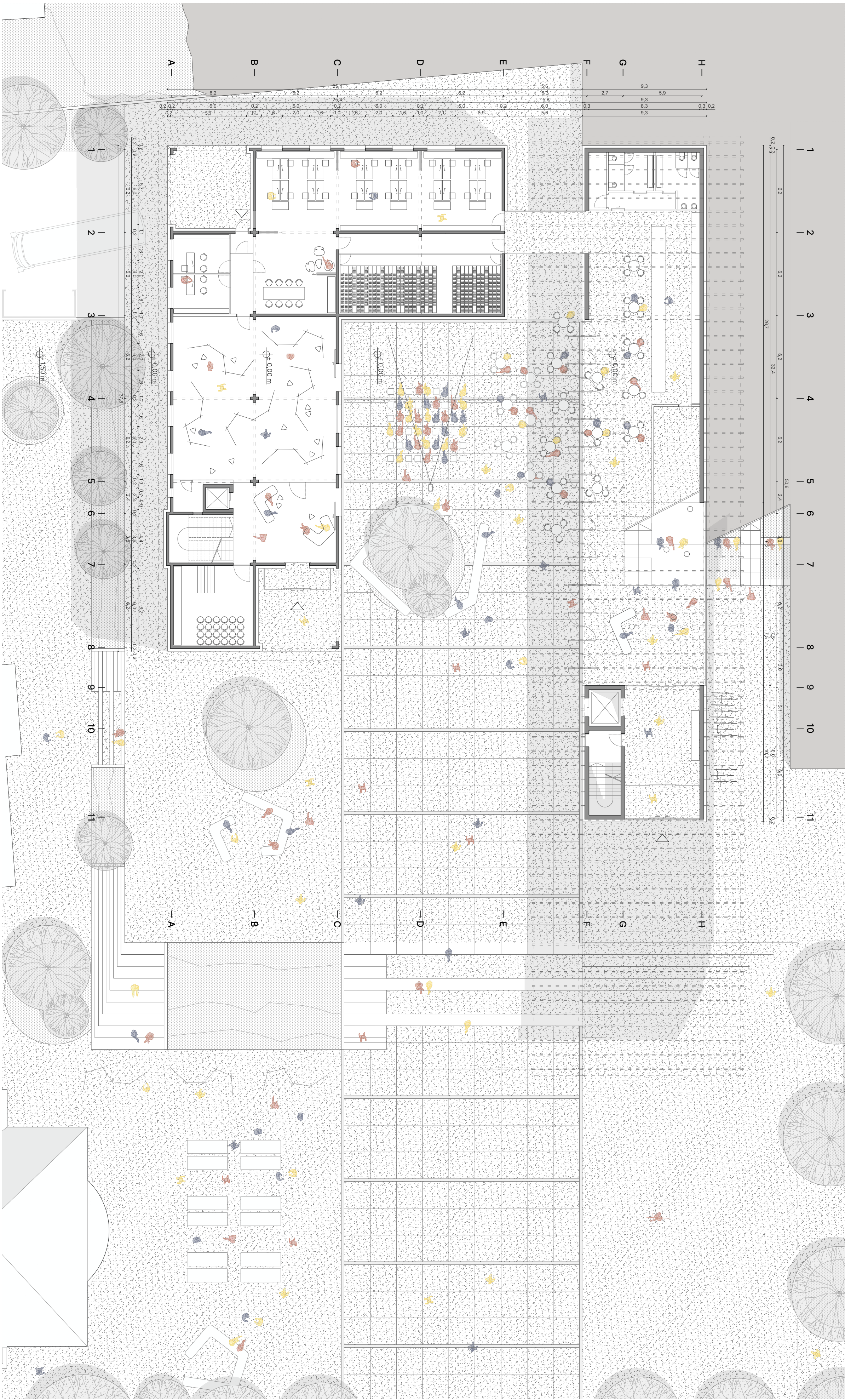
Tloris pritličja, M 1:200
