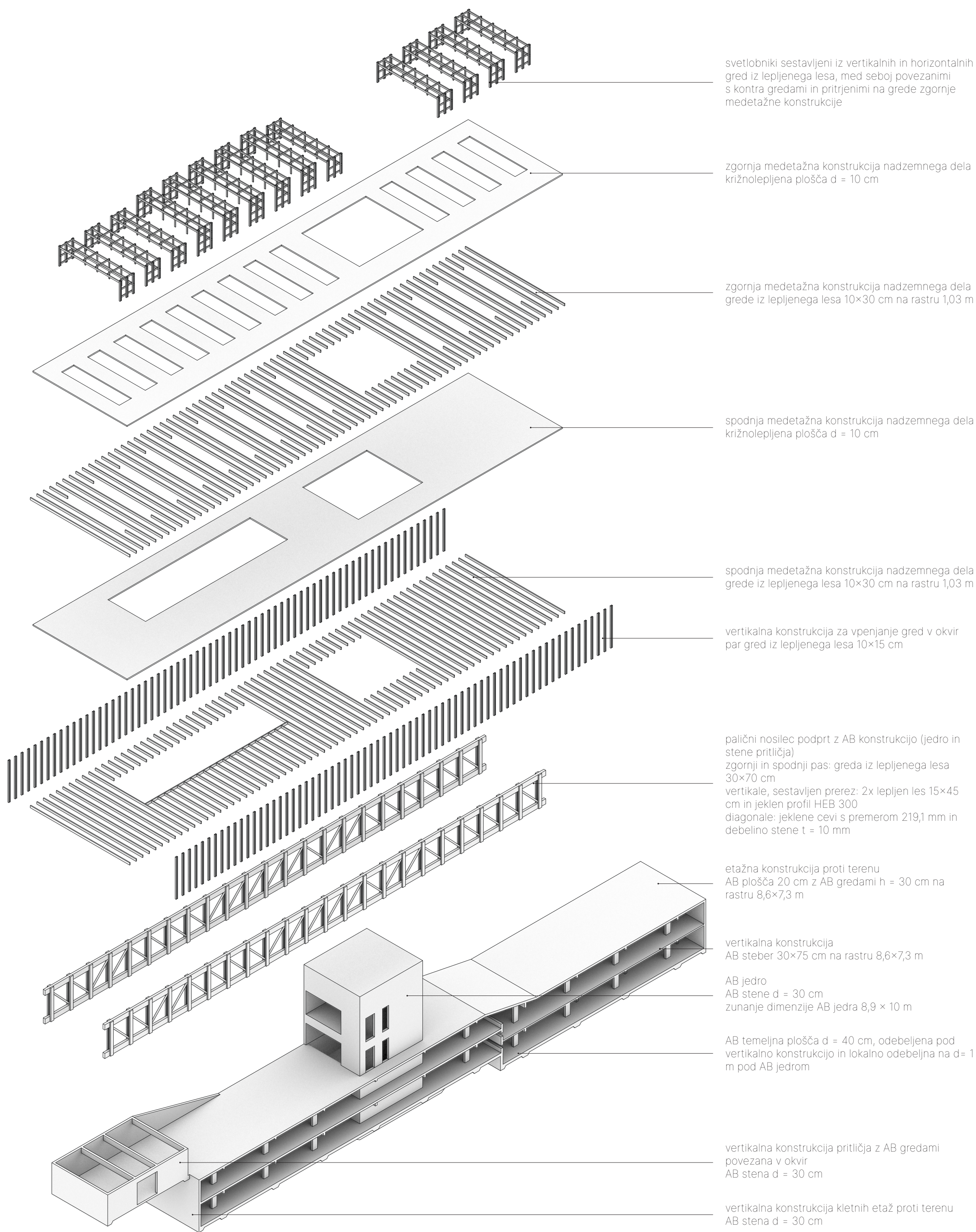
Aksometrični prikaz konstrukcijske zasnove
