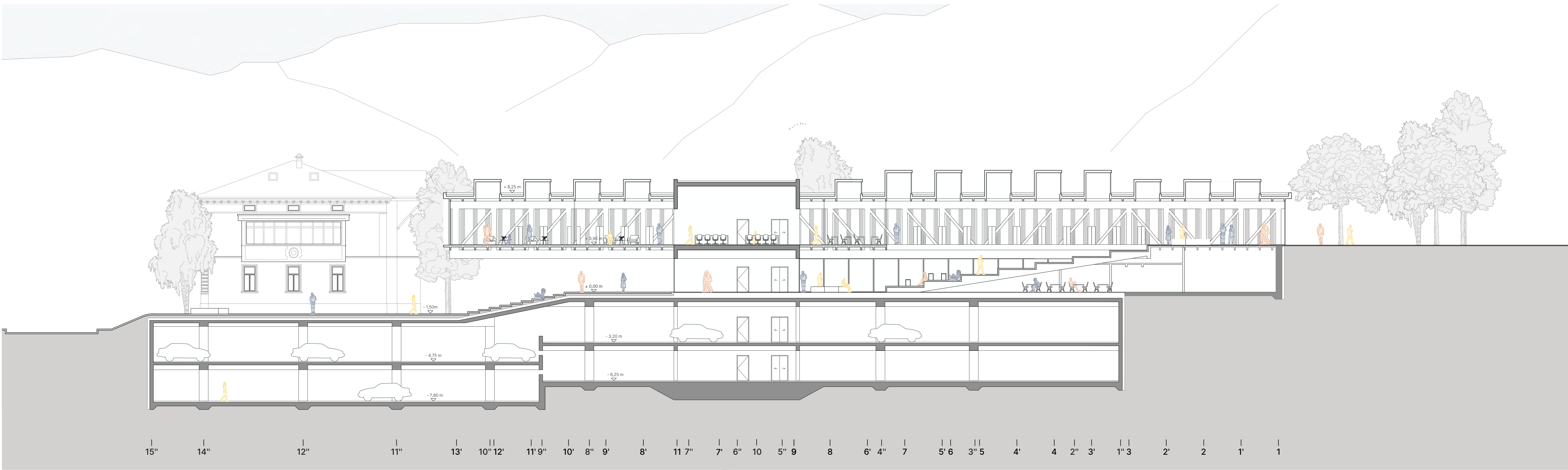
Vzdolžni prežez B-B, M 1:200
