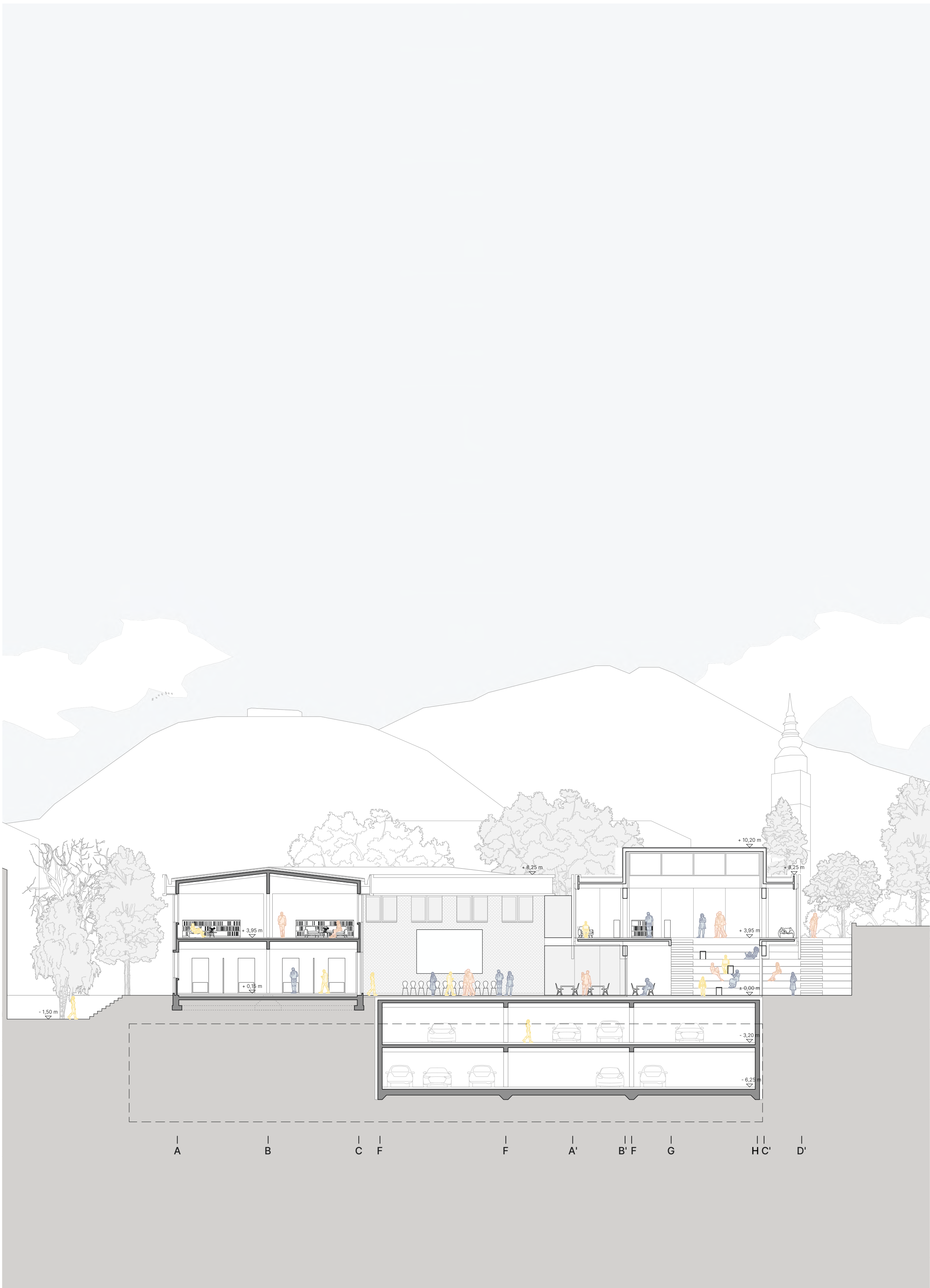
Prečni prerez A-A, M 1:200
