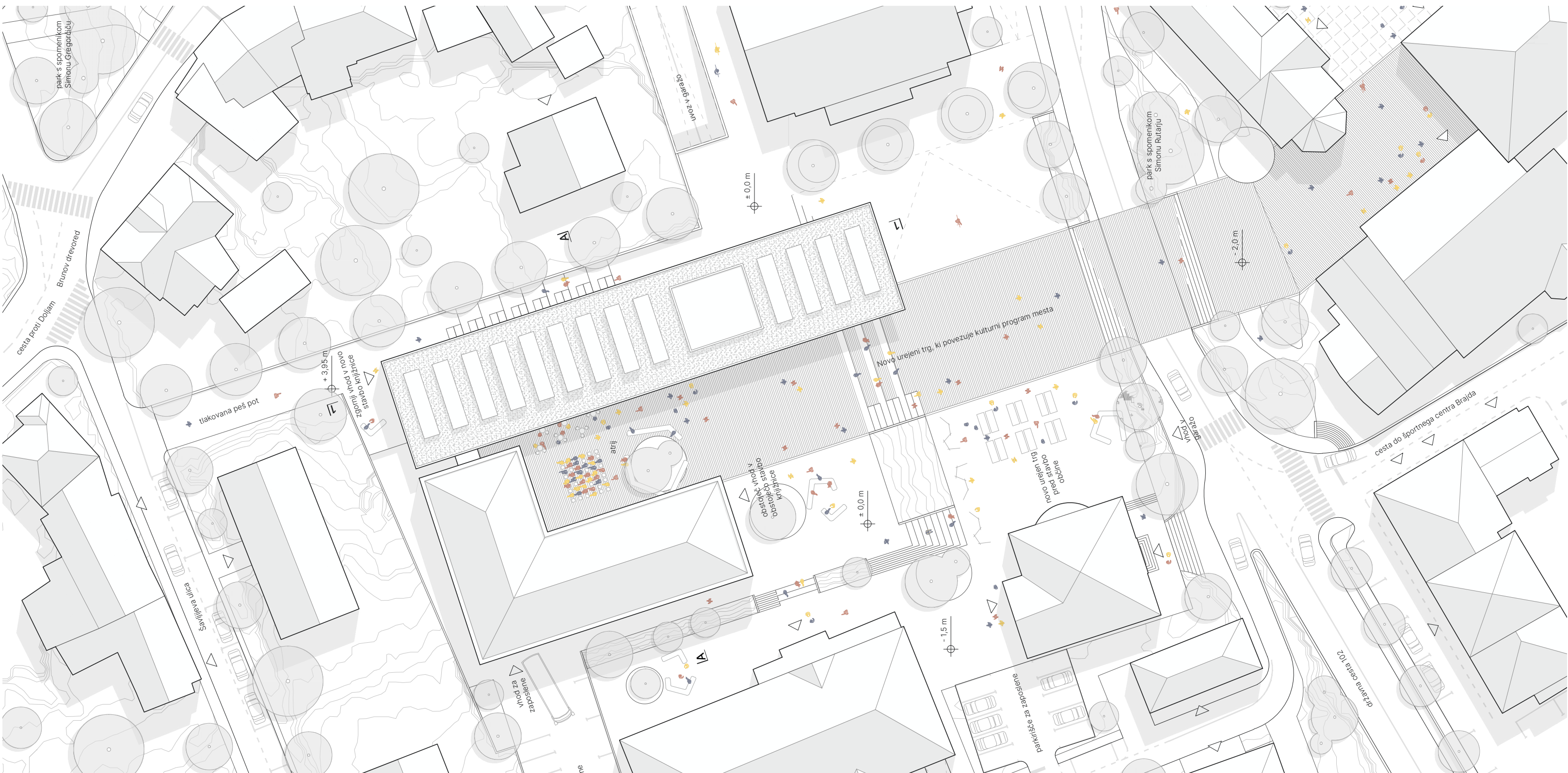
Situacija, M 1:500
