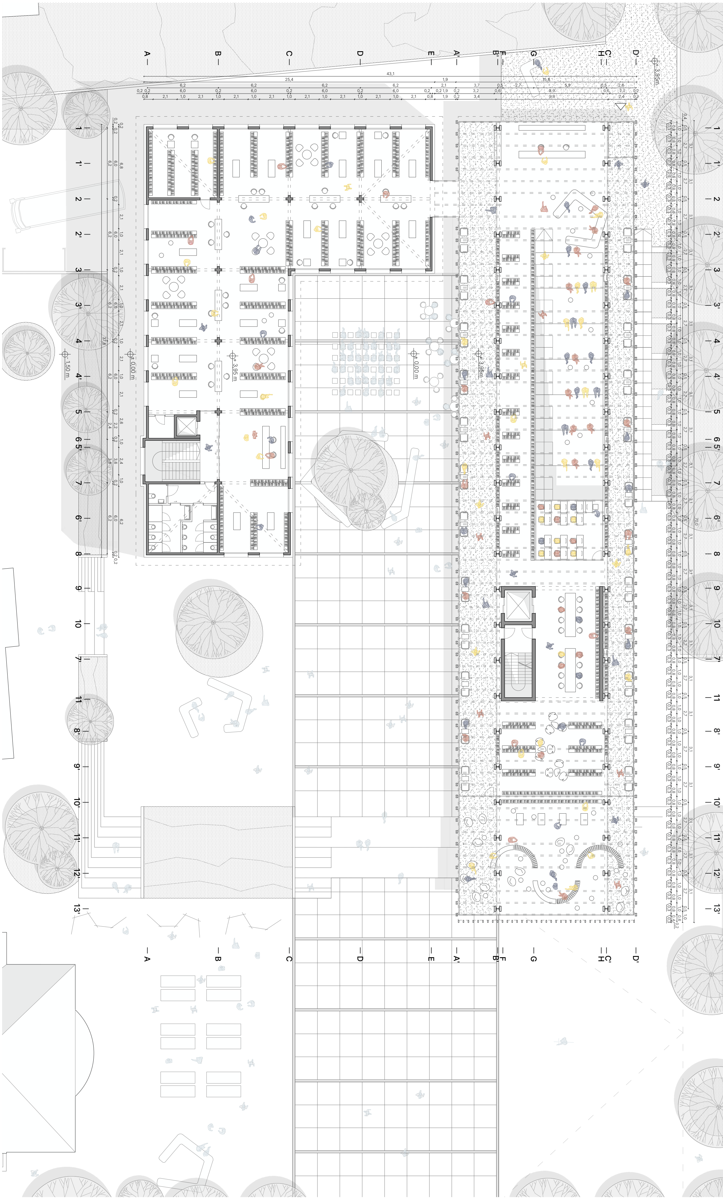
Tloris nadstropja, M 1:200
