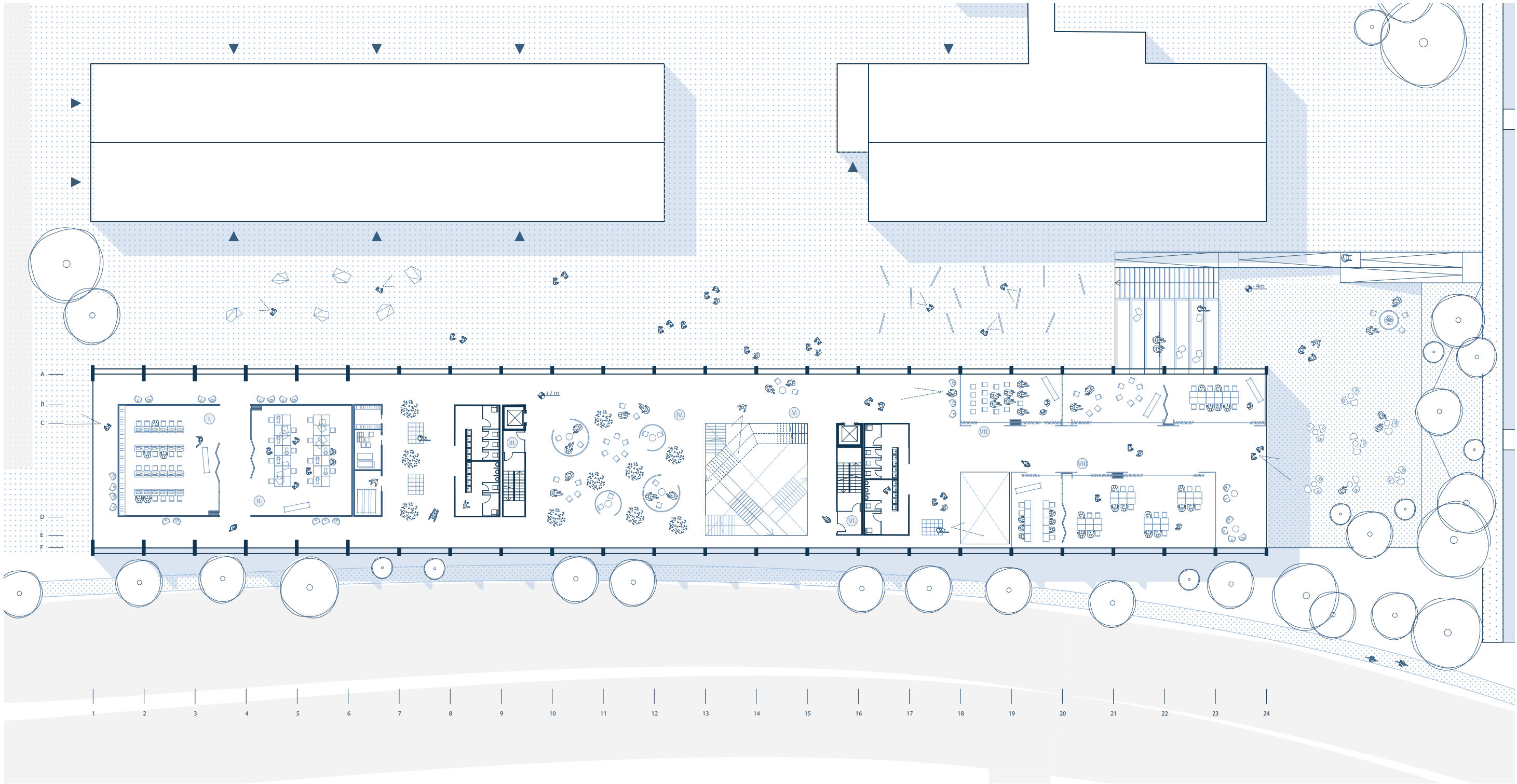
Tloris 2. nadstropja
