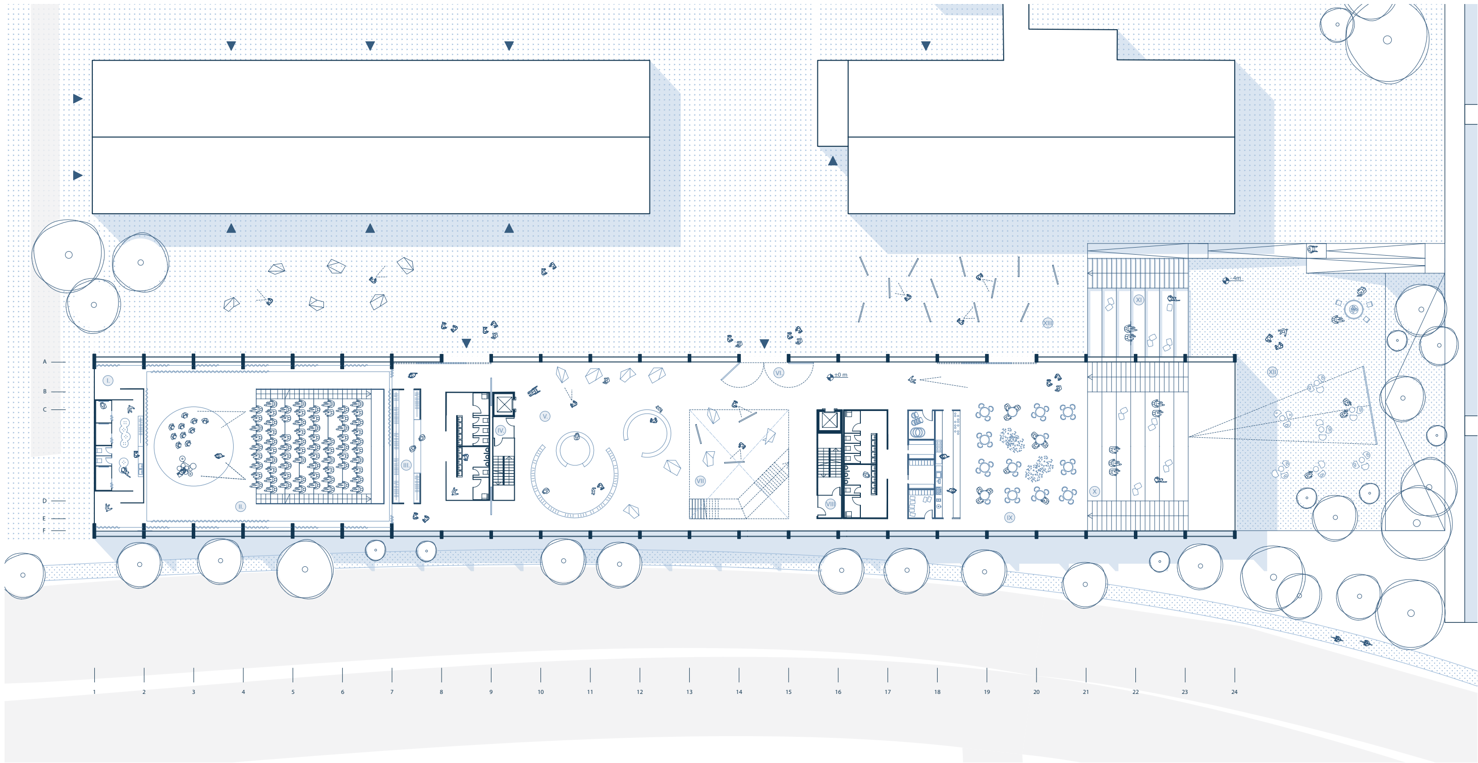
Tloris pritličja
