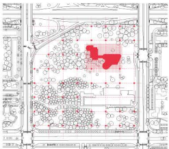
FAZA 3 - Z nadaljnjim zapolnjevanjem polj nastajajo drugi objekti. Volumni objektov so med seboj povezani s koridori širine enega polja.
