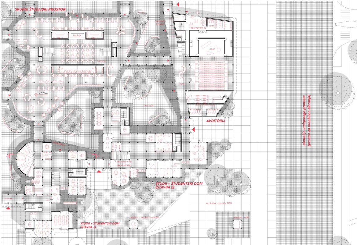
izsek situacije javnega kampusa
