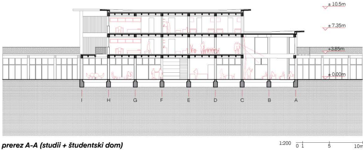
prerez A-A (studij + študentski dom)
