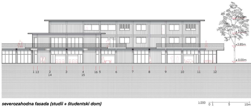
severozahodna fasada (studij + študentski dom)
