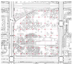
FAZA 1 - Znotraj mreže so določene glavne osi z razdaljo 48 metrov. Polja na križiščih osi so zapolnjena s paviljoni velikosti 4x4m, ki služijo kot referenčne točke za morebitno širitev.
