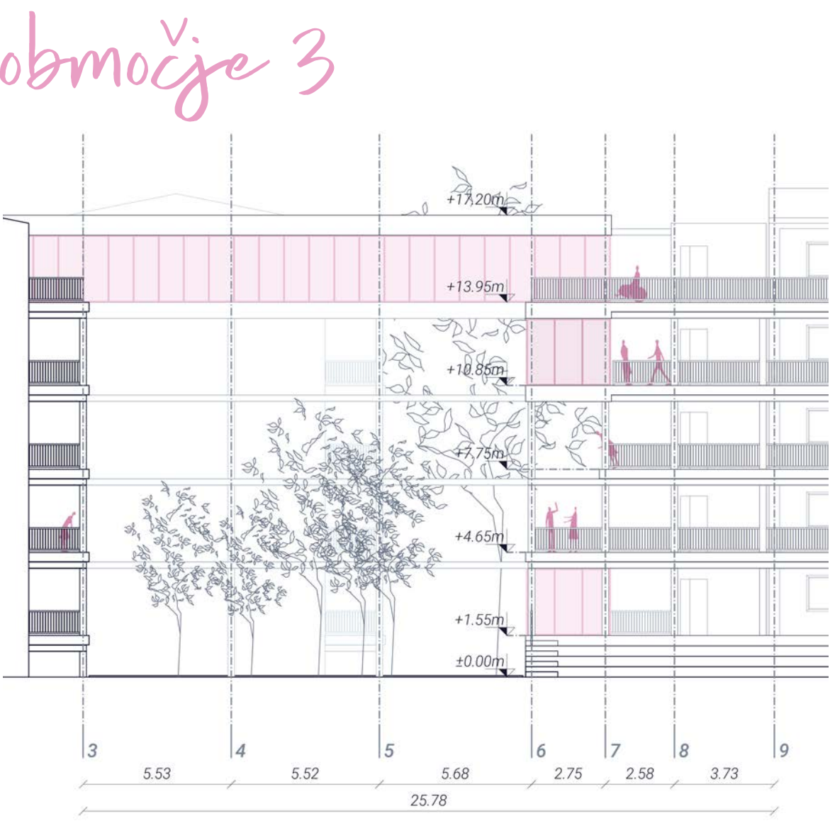
fasada zahod | M 1:200
