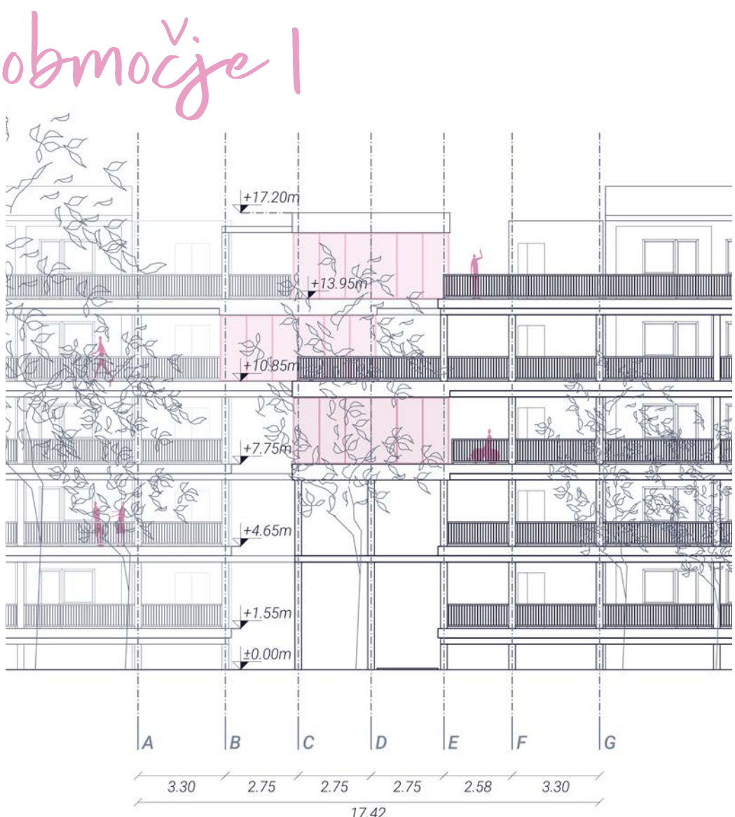
fasada jug | M 1:200
