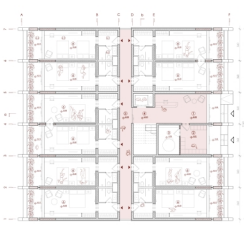
paviljonske hiše | 1. tloris pritličja | M 1:200
