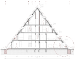
paviljonske hiše | prerez A-A | M 1:200
