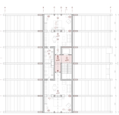
paviljonske hiše | 1. tloris 3. nadstropja | M 1:200
