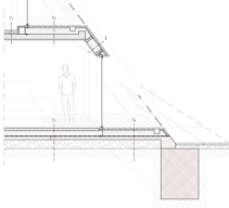
paviljonske hiše | detajl fasadnega pasa | M 1:50
