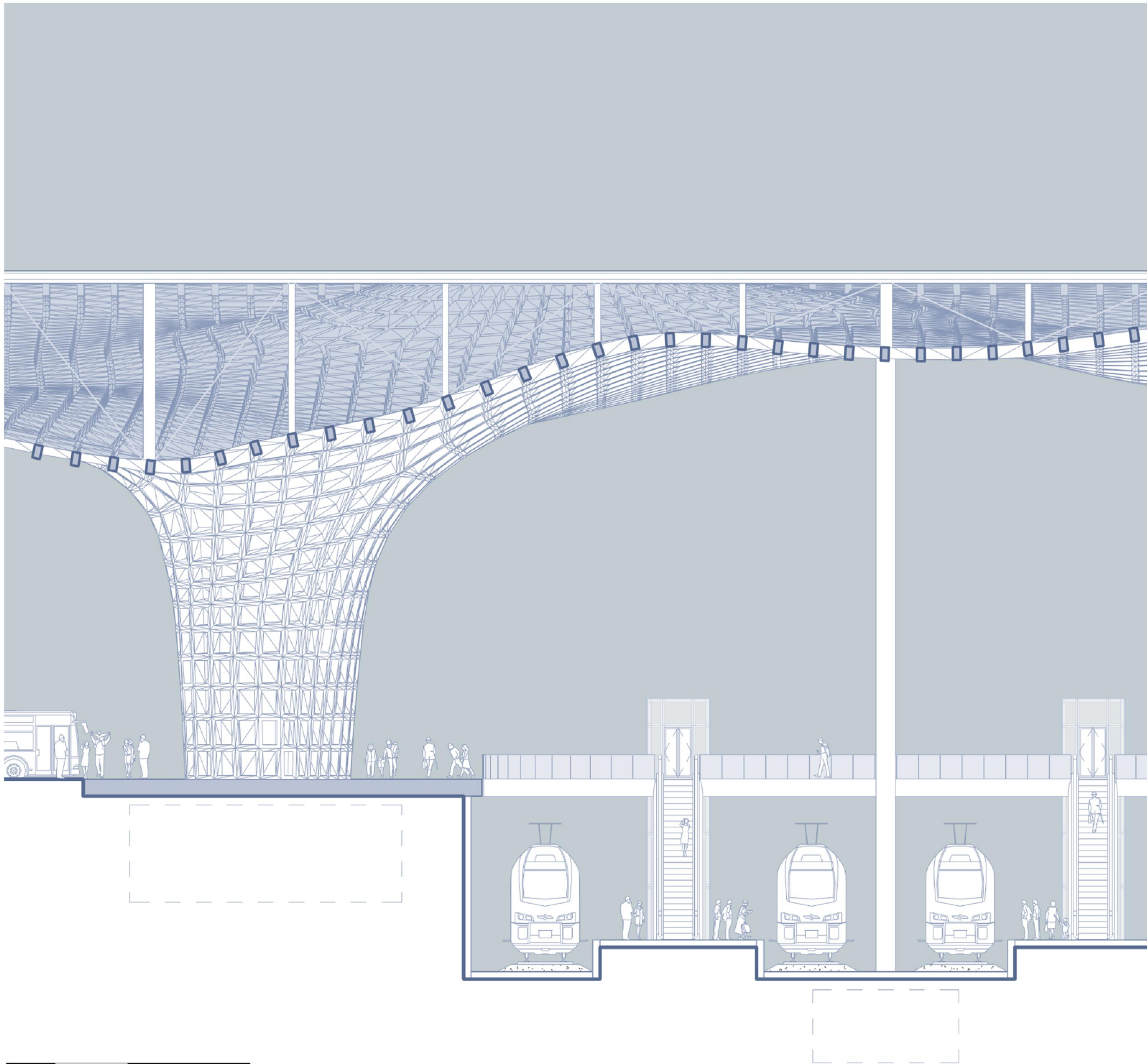
Izsek prereza A - A / M 1:200
