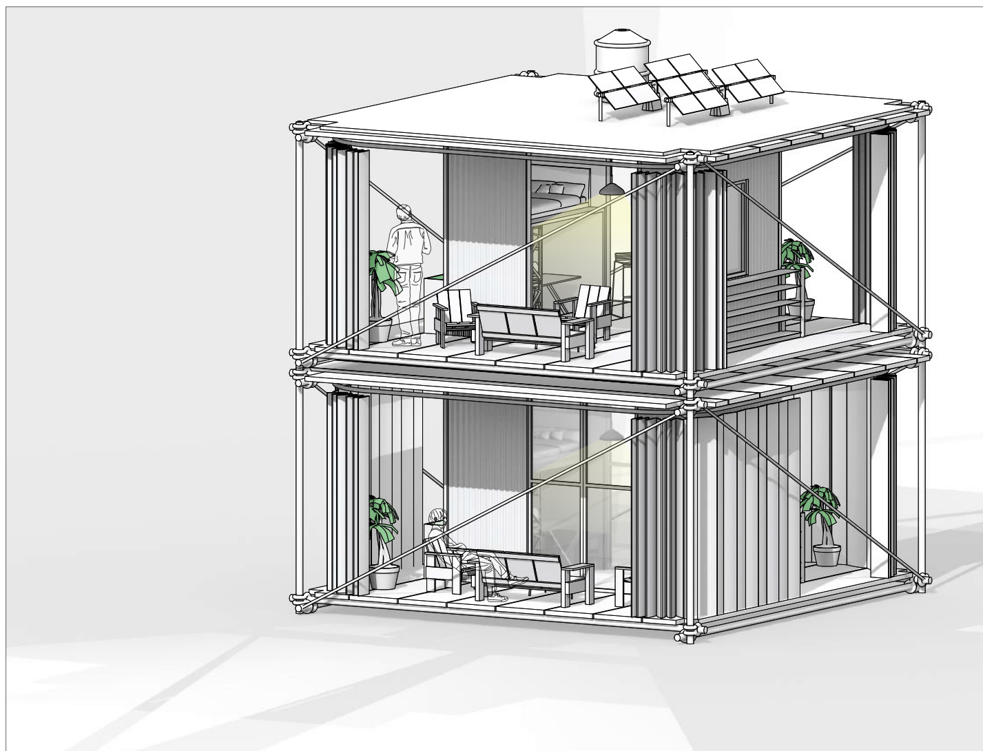
Aksonometrija sestavljenih objektov
