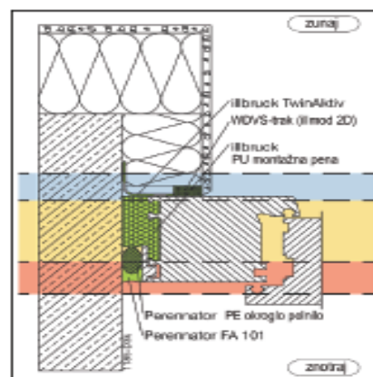
Opcija TwinAktiv in standardnega sistema
