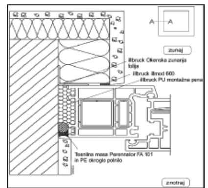
Skica opcije standardnega i3 sistema
