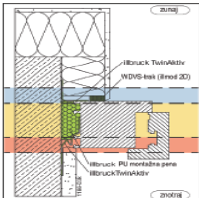
Opcija TwinAktiv sistema
