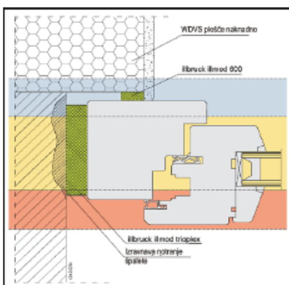
Skica opcije Trioplex sistema
